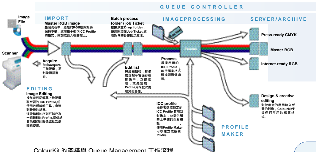
ColourKit 的架構與 Queue Management 工作流程
